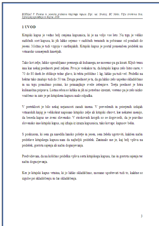
Slika 7: Primer uvoda
